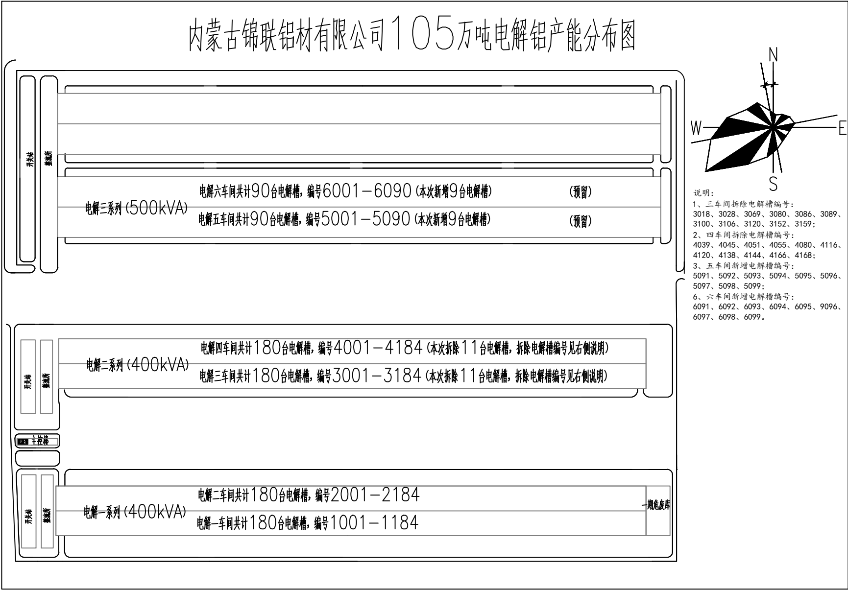
附件3：电解槽产能分布图
